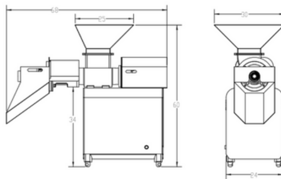
Separador ProMax 1000
